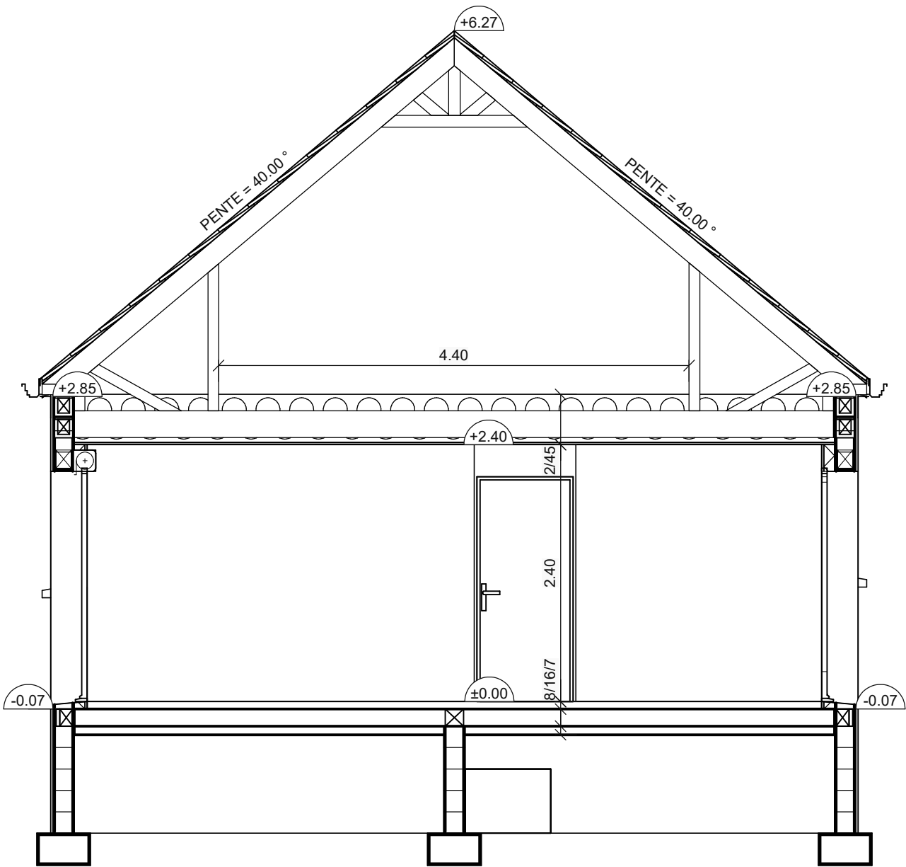
Coupe AA
